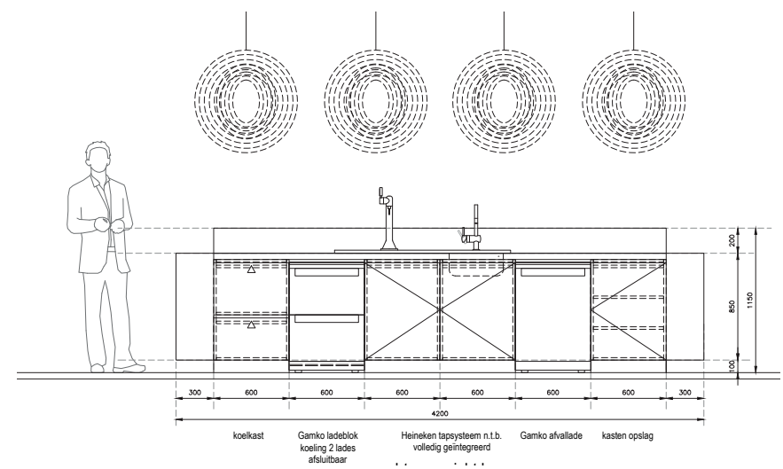
Rechter zij aanzicht
