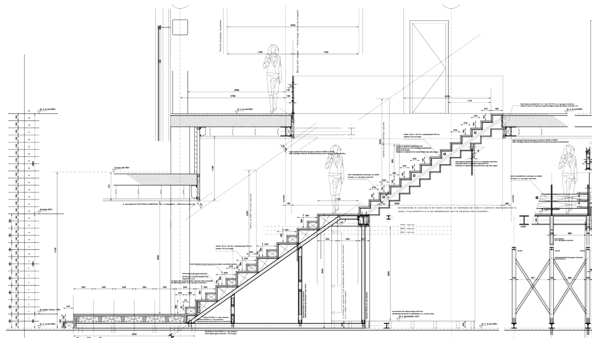
Doorsnede
